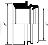
Aknafal csatlakozócsok
