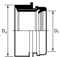
Aknafal-csatlakozócsonk
