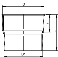
KG 2000 PP átmeneti idom vascsőhöz
