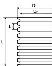
Aknafalcső DN600 – 2 ≤ SN < 4 kN/m 2
