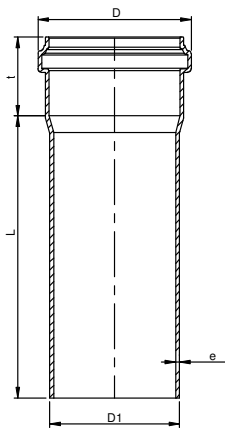
KG 2000 PP csatornacső
