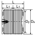
X-Stream PP kettős karmantyú*
