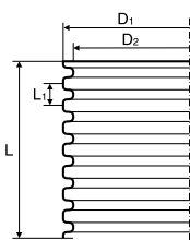
Aknafalcső DN600 – SN ≥ 4 kN/m 2
