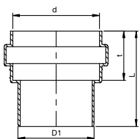
KG 2000 PP átmeneti idom kőagyag csőhöz – csővégre*
