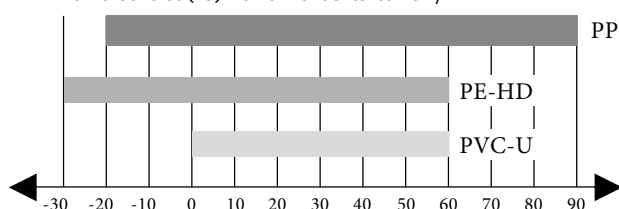
Hőmérséklet (°C) – alkalmazási tartomány
