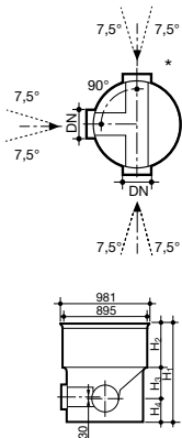
Tegra 800 aknafenek – oldalbekötő
