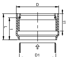
KG 2000 PP átmeneti idom kőagyag csőhöz – tokba*
