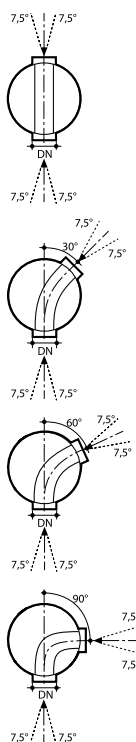
Tegra 800 aknafenek – átfolyós és iránytörő
