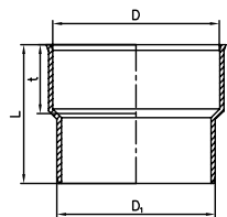
KGUG átmeneti idom acélcsőhöz*
