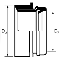
Aknafal csatlakozócsonk
