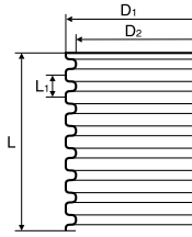
Aknafalcső DN400 – SN ≥ 4 kN/m 2
