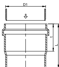
KG 2000 PP átmeneti idom betoncsőhöz*
