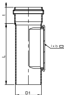
KG 2000 PP tisztítónyílás
