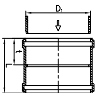
KGMM kettős karmantyú
