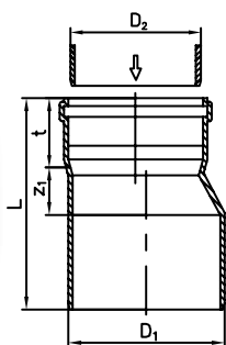
KGR szűkítő
