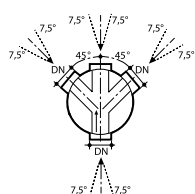
Tegra 1000 NG aknafenek – elágazó 45°
