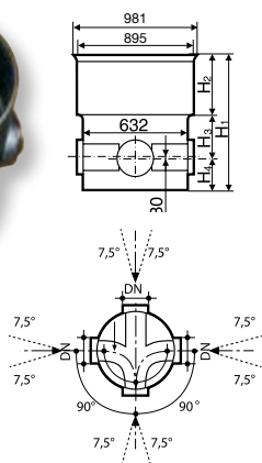
Tegra 800 aknafenek – elágazó 90°
