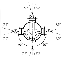
Tegra 1000 NG aknafenek – elágazó 90°
