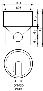
Tegra 800 aknafenek – végakna
