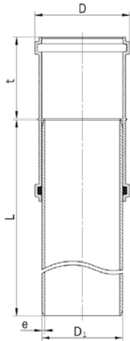
Acaro PP SN 12 csatornacső – kettős karmantyús kötással
