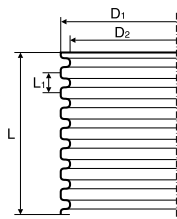
Aknafalcső DN800 – SN ≥ 4 kN/m 2
