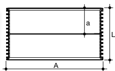
Tegra 600 aknafalcső toldódídom – 2 db gumigyűrűvel
