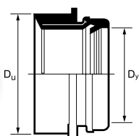
Tegra 1000 NG PVC aknabekötő idom
