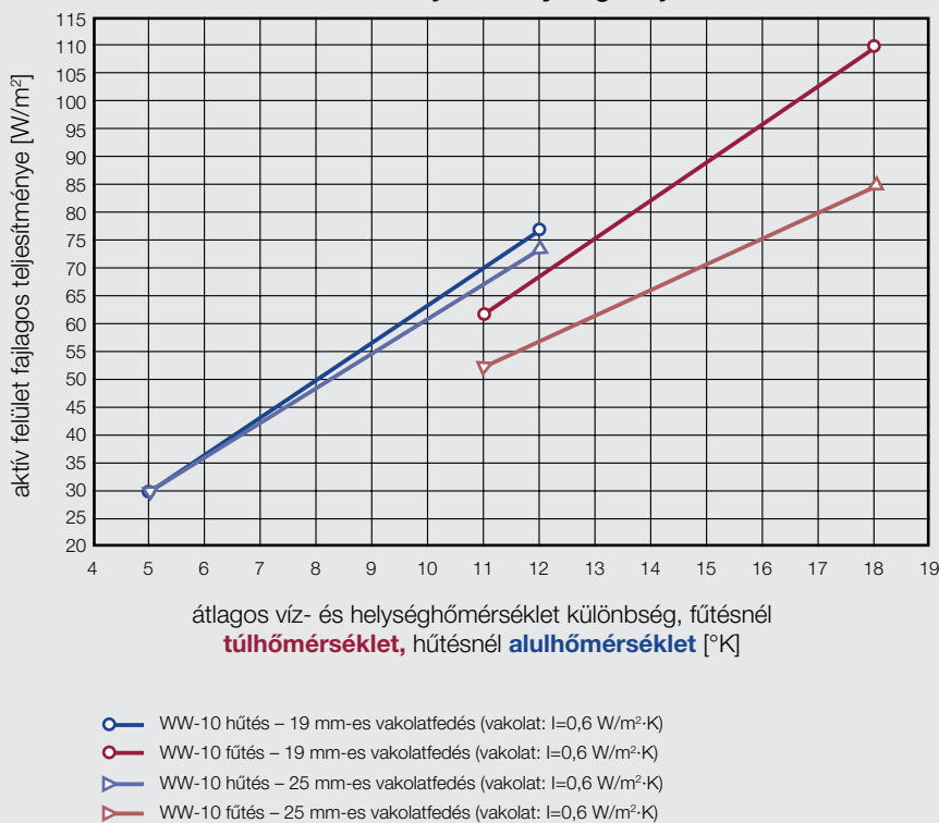
Wavin Tempower WW-10 felületfűtési -hűtési rendszer teljesítménydiagramja
