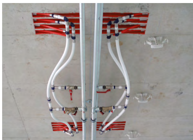
A födém a zsaluzat eltávolítása után a mennyezet alatt vezetett gyűjtővezetékekkel és a bekötött CW-90 panelokkal
