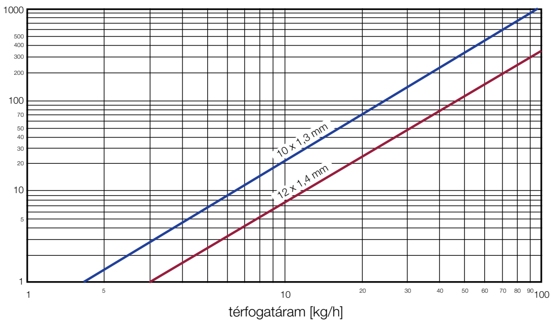
Wavin Tempower WW-10 nyomásvesztés diagramja 10x1,3 mm-es és 12x1,4mm-es rendszercső átmérőnél
